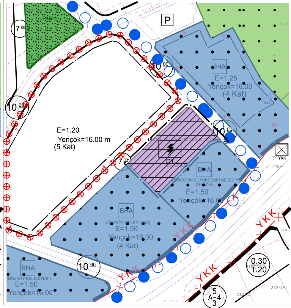
ÖNERİ PLAN
